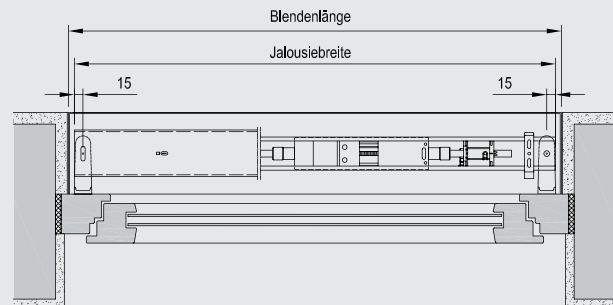
Horizontalschnitt EL 80 S
