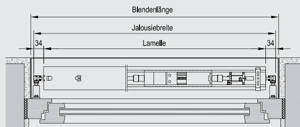
Horizontalschnitt EL 80 NF
