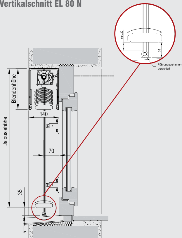
Vertikalschnitt EL 80 N
