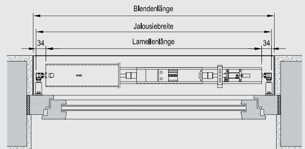
Horizontalschnitt EL 80 N
