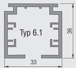
Oberschiene
