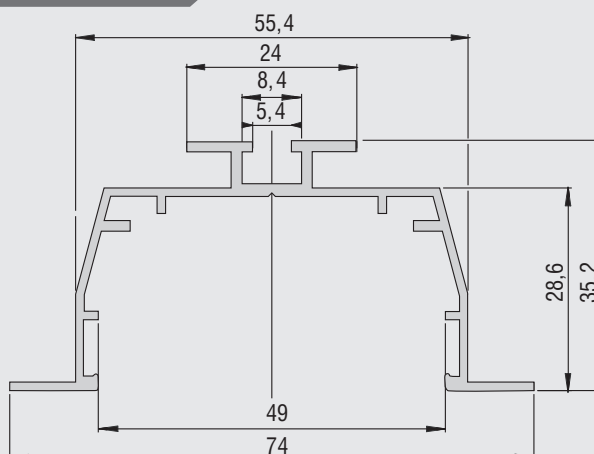
Einbauprofil mit Halterbefestigung (abgehängte Decke) - 7 m Länge
