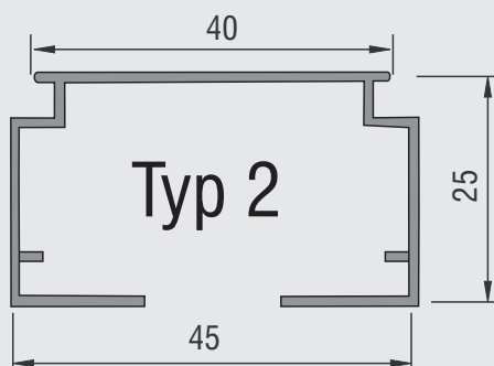
Einbauprofil mit Halterbefestigung (abgehängte Decke) - 7 m Länge
